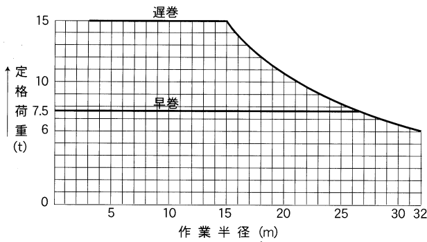
【定格荷重線図】
