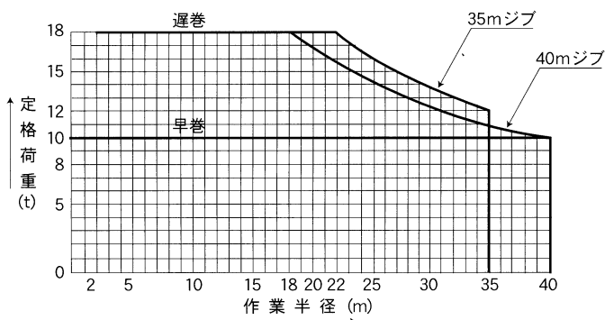
【定格荷重線図】
