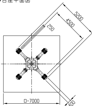
● 台座平面図
