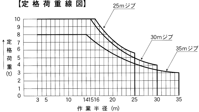
【定格荷重線図】
