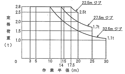
定格荷重線図
