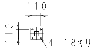
ベース詳細図
