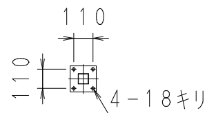
ベース詳細図
