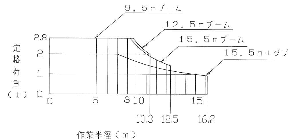
性能曲線図
