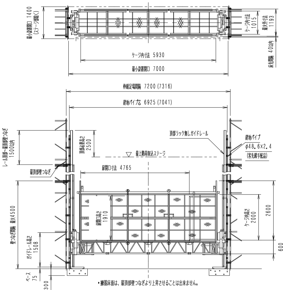
【ベース平面図】
