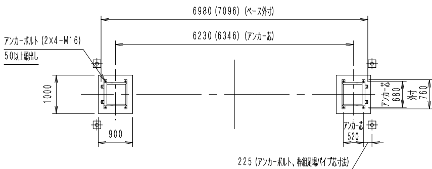
【ベース平面図】
