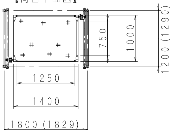
【荷台平面図】
