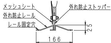
A-A断面図
