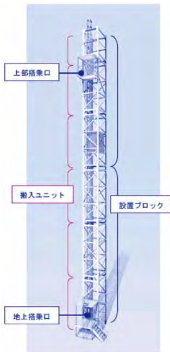
ユニット化されたエレベータシャフト
